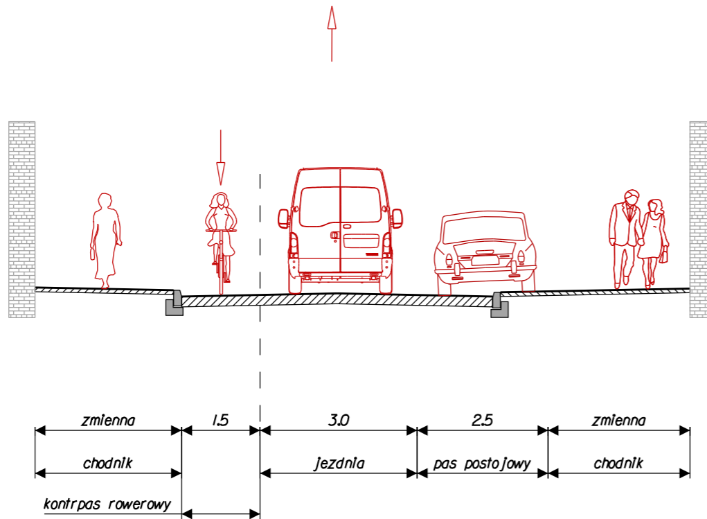
Przekrój ul. Wiatrakowej (wlot na skrzyżowanie z ul. Nowodworską)
